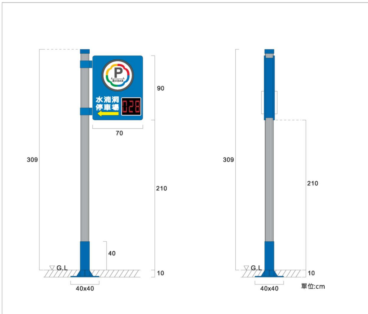
立面圖
